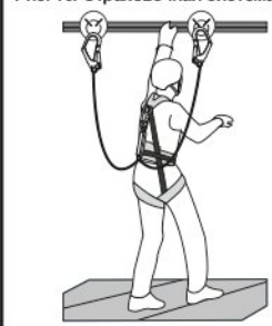
Рис. 10. Страховочная система
