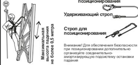
Рис. 14. Позиционирование в рабочем положении
