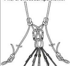
Рис. 5. Способы крепления
