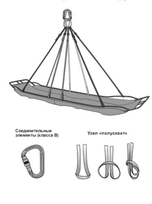
Рис. 3. Использование подвесной системы «Спайдер»
