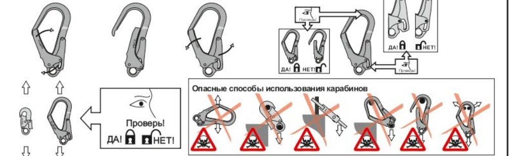
Рис. 6. Краткая пиктографическая информация по использованию карабинов, входящих в комплектацию стропов.
