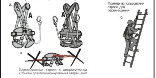
Рис. 6. Краткая пиктографическая информация по использованию карабинов, входящих в комплектацию стропов.
