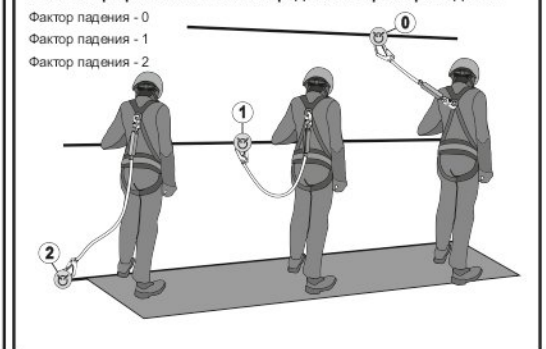
Рис. 10. Графическая схема к определению фактора падения
