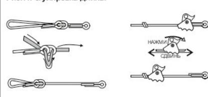
Рис. 7. Регулировка длины
