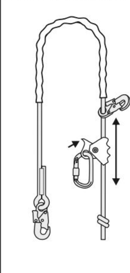
Рис. 6. Регулировка длины стропа
