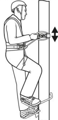
Рис. 7. Рабочее положение
