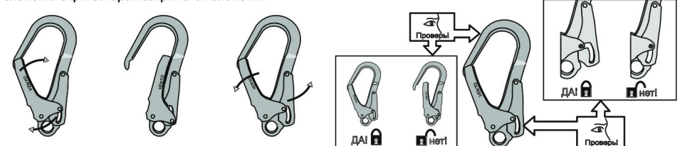
Рис. 5. Открытие / закрытие самозапирающегося запорного элемента с фиксатором закрытого положения
