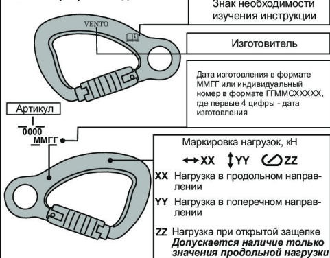
Рис. 2. Маркировка изделий
