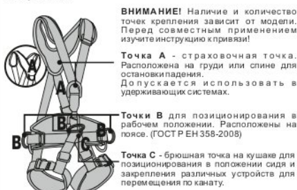
Рис. 3. Расположение и назначение крепёжных точек на привязях
