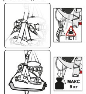
Рис. 14. Способ интеграции рабочего сидения
