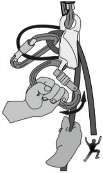
Рис. 15. Разблокировка устройства
