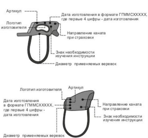
Рис. 2. Маркировка изделия
