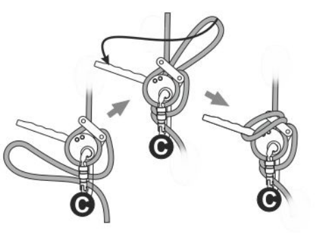
Рис. 13. Блокировка устройства
