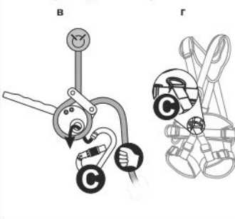
Рис. 8. Спуск груза
