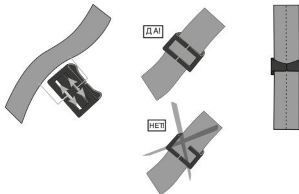
Рис. 5. Правильная установка скобы на ленте
