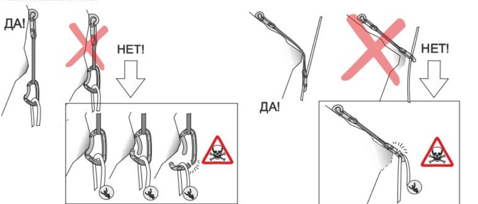
Рис. 6. Установка оттяжек
