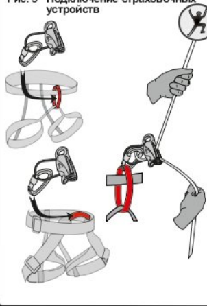
Рис. 5. Подключение страховочных устройств
