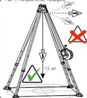
Рис. 9 Направление нагрузки
