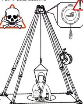
Рис. 8 Безопасность
