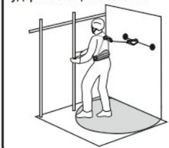
Рис. 11. Способ организации удерживающей системы
