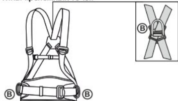
Рис. 2. Типы крепежных точек
