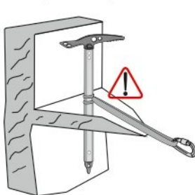
Рис. 7. Т-образная станция
