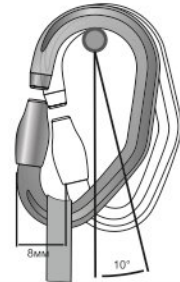
Рис. 6. Допустимый угол отклонения карабина при нагрузке
