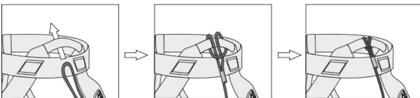
Рис. 5. Крепление усов
