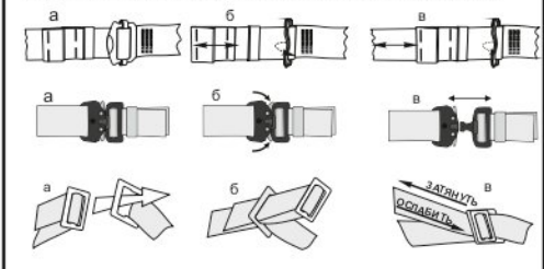
Рис. 7. Типы используемых пряжек, способы заправки
