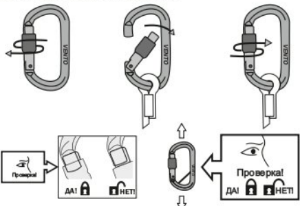
Рис. 3. Использование карабинов
