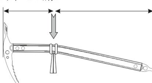
Рис. 8. Центр тяжести ледоруба
