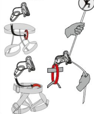
Рис. 8. Блокировка грудной обвязки и поясной беседки
