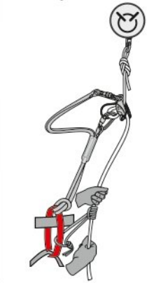
Рис. 9. Подключение к веревке
