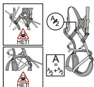
Рис. 11. Использование полных обвязок
