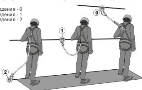
Рис. 13. Графическая схема к определению фактора падения
