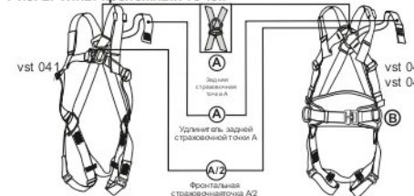
Рис. 2. Типы крепежных точек
