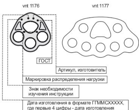
Рис. 1. Общий вид и маркировка изделия
