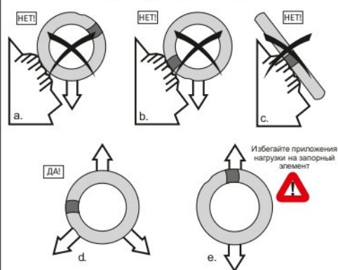
Рис. 3. Приложение нагрузки к разъемному кольцу
