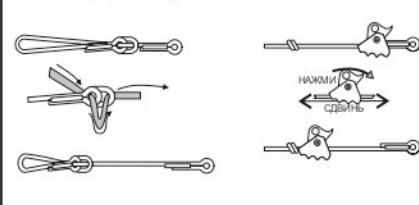
Рис. 7. Регулировка длины
