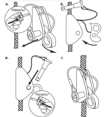
Рис. 3. Установка зажима на канат
