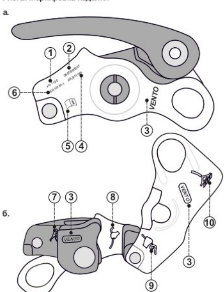
Рис. 2. Маркировка изделия
