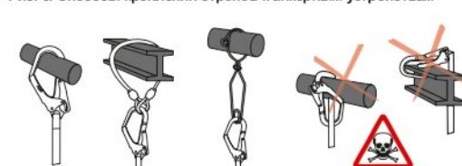
Рис. 6. Способы крепления стропов к анкерным устройствам
