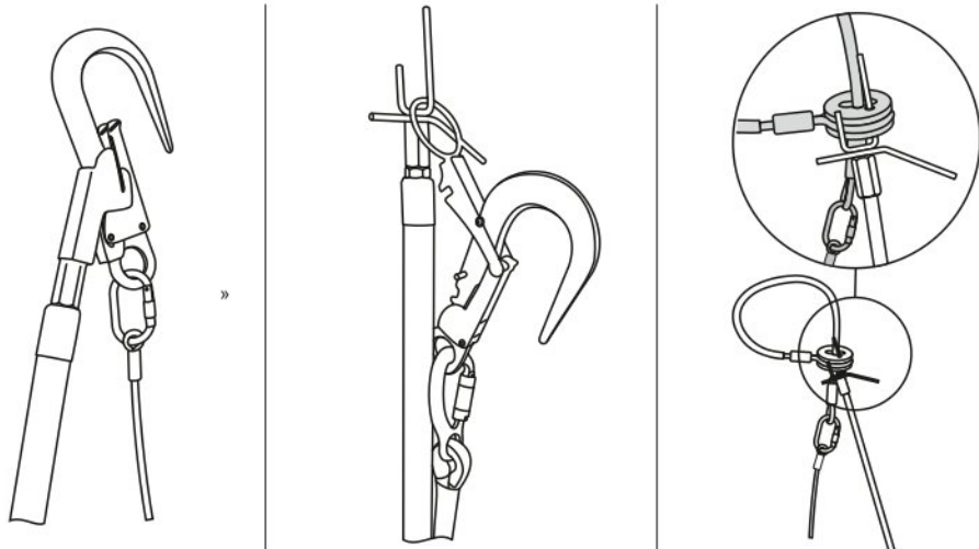
Рис. 3. Примеры использования наконечников с различными анкерными устройствами
