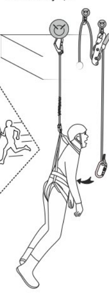
Рис. 3д. Перережьте строп
