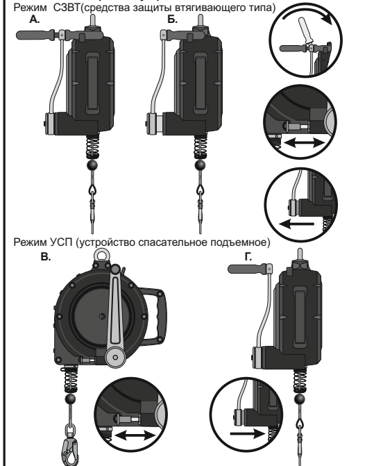
Рис. 6. Режимы работы устройства «НВ evak»
