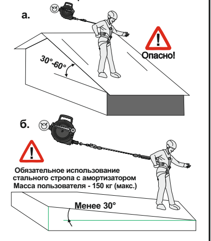
Рис. 9. Использование на горизонтальных и наклонных поверхностях
