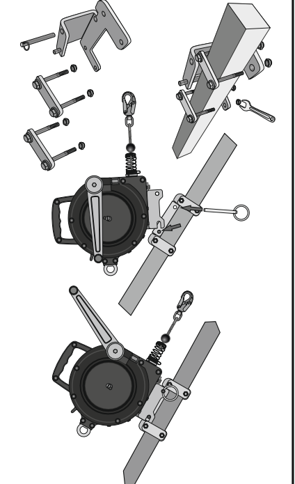
Рис. 9. Использование на горизонтальных и наклонных поверхностях
