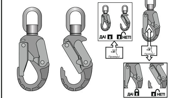
Рис. 5. Общие принципы использования карабинов
