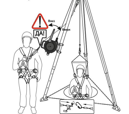
Рис. 8. Использование лебедки совместно с треногой
