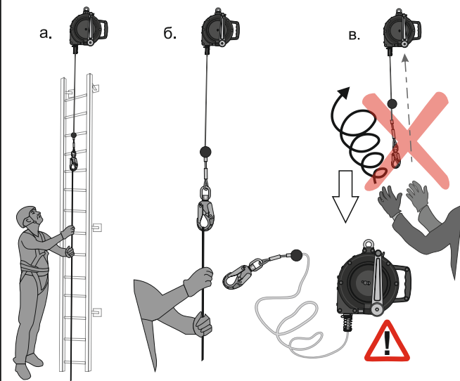
Рис. 13. Использование троса в режиме средства защиты втягивающего типа
