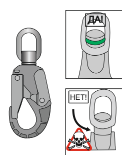
Рис. 15. Проверка индикаторов срыва на карабине
