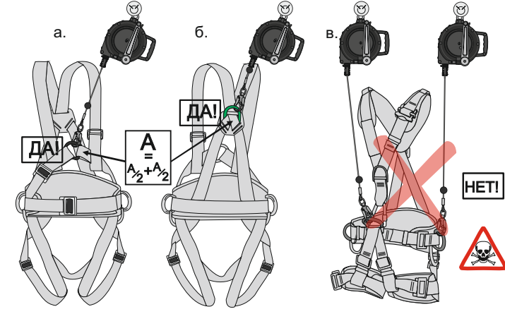
Рис. 5. Общие принципы использования карабинов
