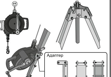
Рис. 7. Способы установки «НВ evak» на треногу при помощи адаптера
