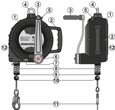
Рис. 1. Внешний вид, составные части и параметры
