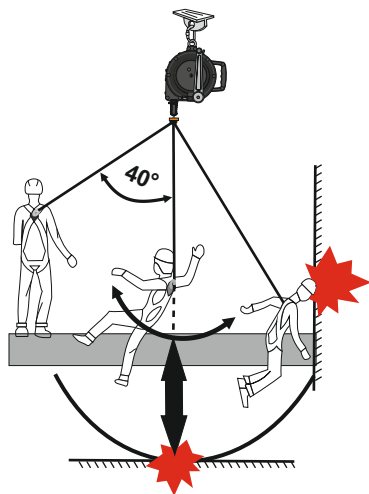
Рис. 11. Ограничения по использованию средства защиты втягивающего типа
