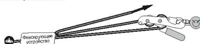
Рис. 14. Простой полиспаст
