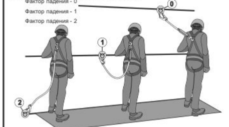
Рис. 11. Использование стропов без амортизатора
