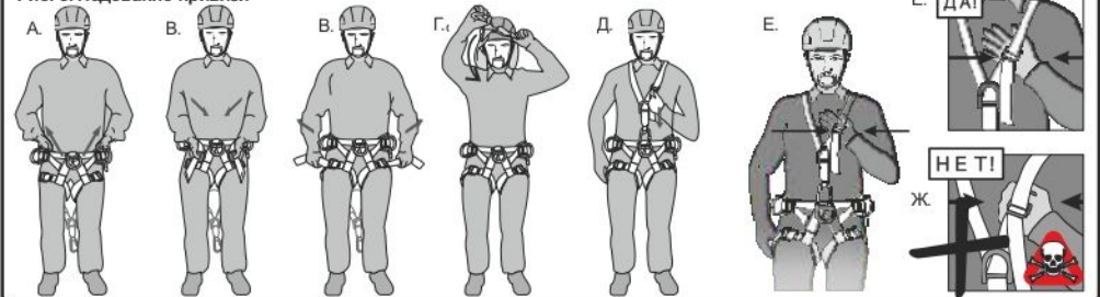
Рис. 8. Надевание привязи
