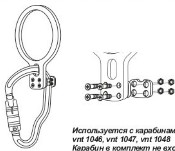
Рис. 4. Установка на беседку
