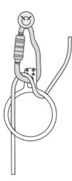
Рис. 5. Установка на точку
