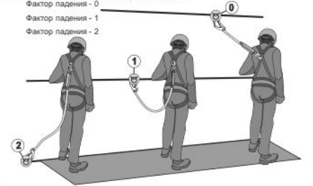
Рис. 11. Использование стропов без амортизатора
