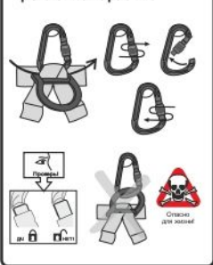
Рис. 12. Страховочная система
