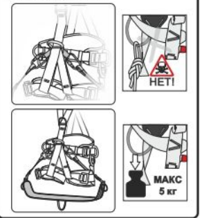
Рис. 14. Способ интеграции рабочего сиденья
