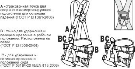
Рис. 3. Маркировка изделия
