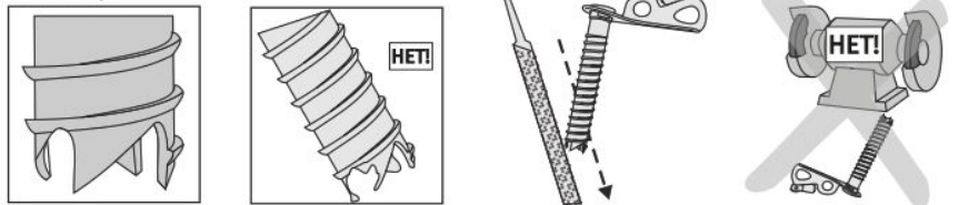
Рис. 12. Заточка коронки
