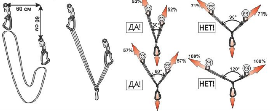
Рис. 5. Организация ледовой проушины (vpro 0183)
