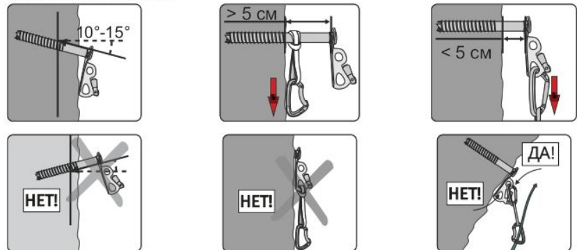
Рис. 7. Положение анкерного устройства
