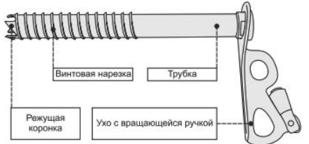
Рис. 2. Идентификация изделия
