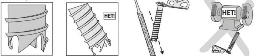
Рис. 12. Заточка коронки
