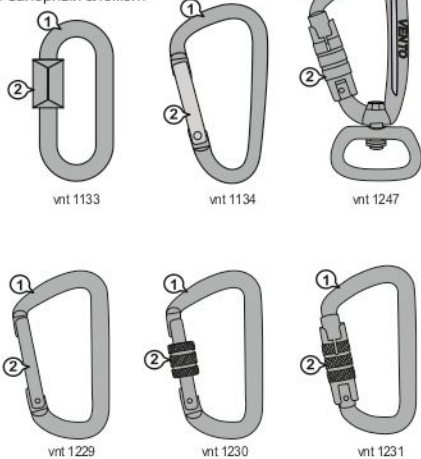
Рис. 1. Общий вид и составные детали
