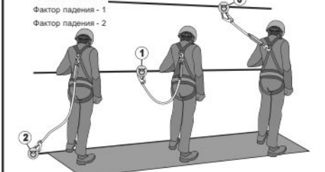
Рис. 11. Использование стропов без амортизатора
