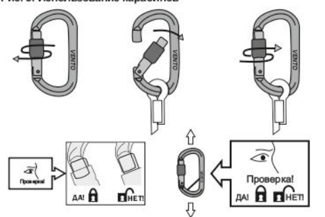
Рис. 3. Использование карабинов
