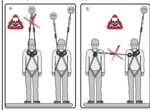
Рис. 12. Ограничения использования двухплечевого «НВ-02»
