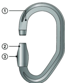
Рис. 2. Маркировка изделия
